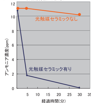
アンモニア吸着濃度低下試験
