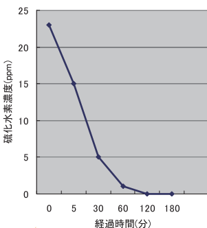
硫化水素(腐敗臭)の濃度低下試験
